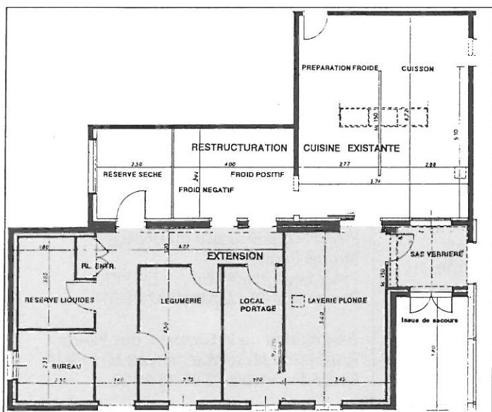
Plan de la cuisine et annexes
