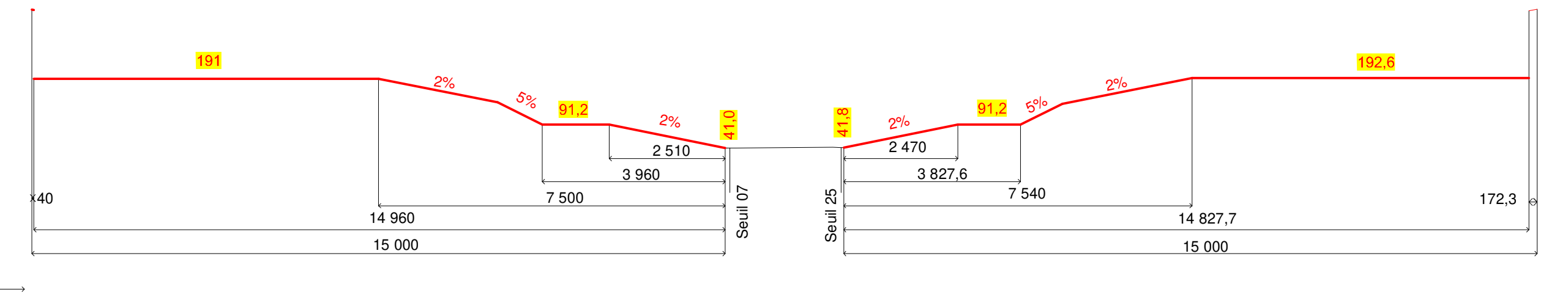
PROFIL EN LONG TYPE PISTE 07-25
