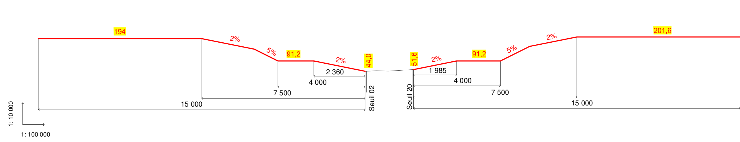
PROFIL EN LONG TYPE PISTE 02-20
