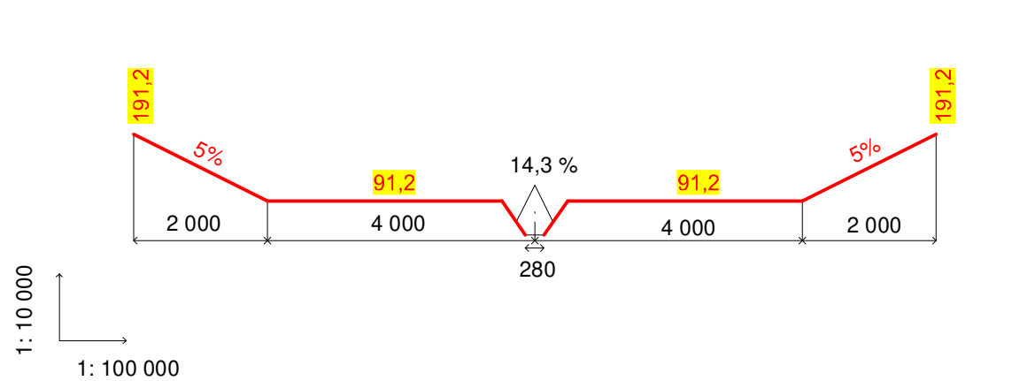
PROFIL EN TRAVERS TYPE AVANT INTERSECTIONS
